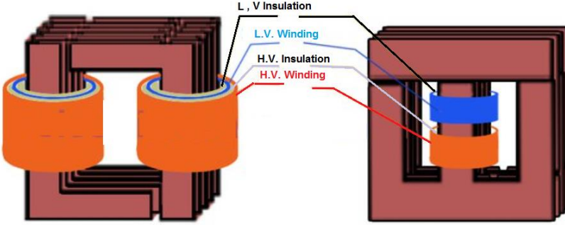
Şekil 2 Çekirdek ve mantel tip transformatörler
