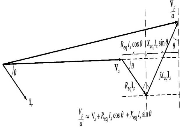
Şekil 13 Transformatörün vektör eşdeğer devresi
