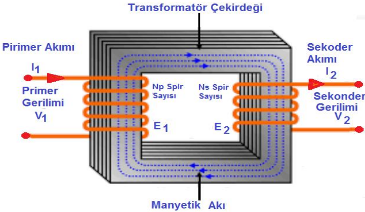
Şekil 1. Bir fazlı transformatörün görünüşü
