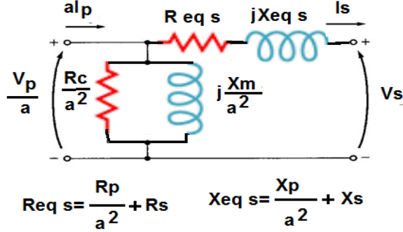
Şekil 10 Transformatörün eşdeğer devresi
