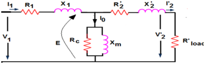
Şekil 7 Bir fazlı asenkron motorun eşdeğer devresi
