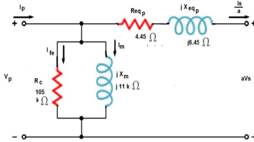
Şekil 14 Transformatörün sekondere indirgenmiş eşdeğer devresi
