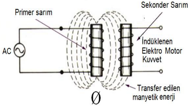
Şekil 6 Transformatörlerde indüklenen gerilim
