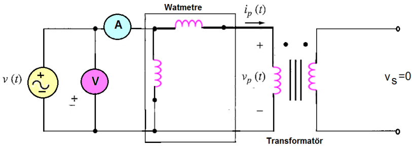
Şekil 7 Bir fazlı transformatörün boştaki çalışması
