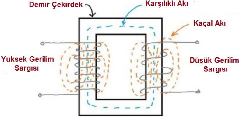
Şekil 8 Transformatör kaçak akıları
