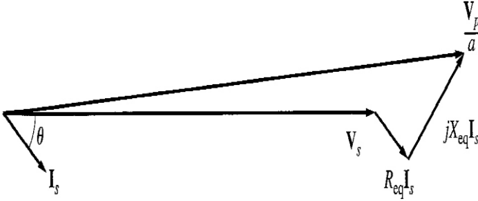
Şekil 11. Geri (Endüktif-Lagging) Power Factor (Güç Faktörü)
