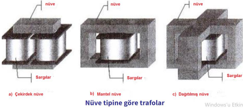
Şekil 4 Nüve türlerine göre transformatörler
