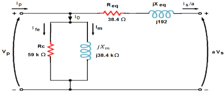
Şekil 9 Bir fazlı transformatörün eşdeğer devresi
