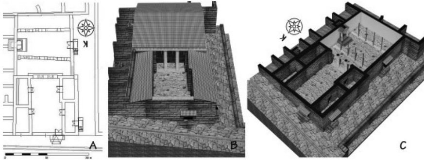
Fig. 14. A. Zemin Kat Planı B. Çatı Planı C. Kat Planı Perspektifi
