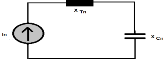
Şekil 14 Güç sisteminin n harmonikteki eşdeğer devresi
