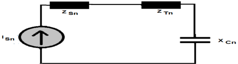
Şekil 15 Güç sisteminin n harmonikteki eşdeğer devresi
