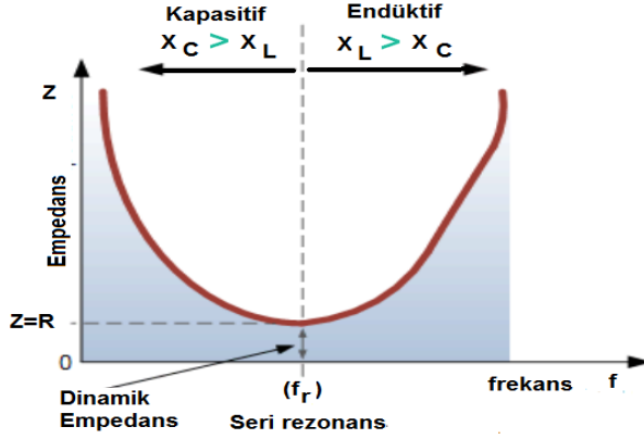
Şekil 6 Seri rezonans devresinde empedans
