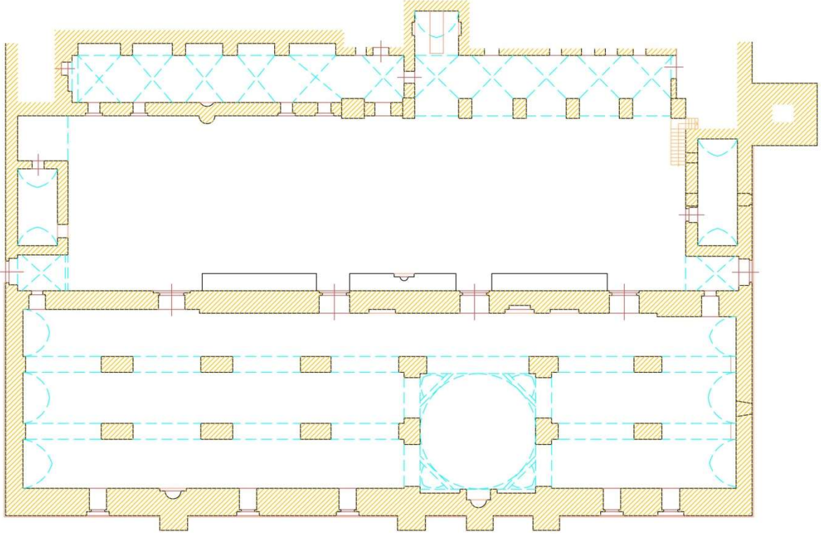
Çiz. 1: Mardin Ulu Cami Vaziyet Planı (A. Gabriel'den işlenerek)
