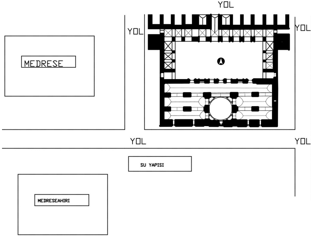
Çiz. 3: Mardin Ulu Cami Külliyesi'nin Vaziyet Planı (Vakfiyeye Göre)
