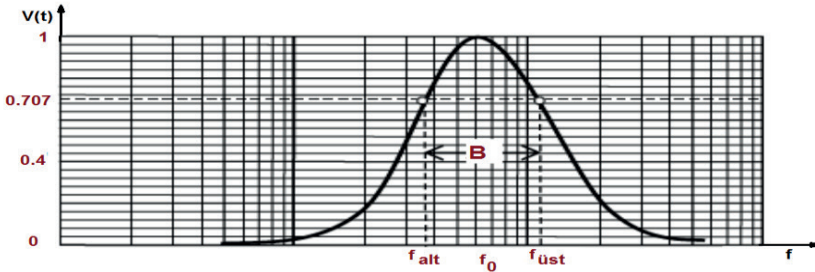
Şekil 5 Paralel rezonans devresinde gerilimin frekansa göre değişimi
