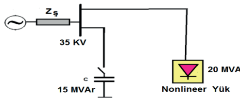
Şekil 7. Güç sisteminin prensip şeması
