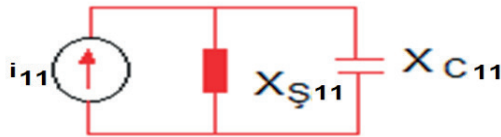
Şekil 10. Onbirinci harmonik bileşen için eşdeğer devre
